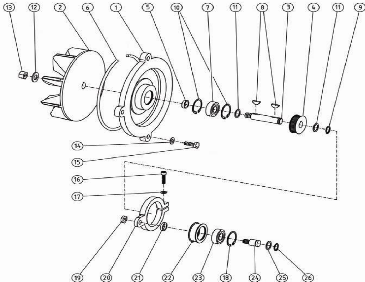
Bona Universal AMO110013.0 Universal ventilator
