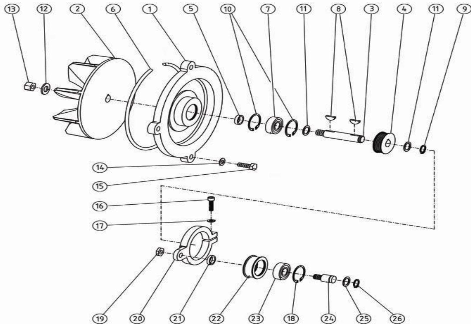
Bona Universal AM0001503 Universal ventilator
