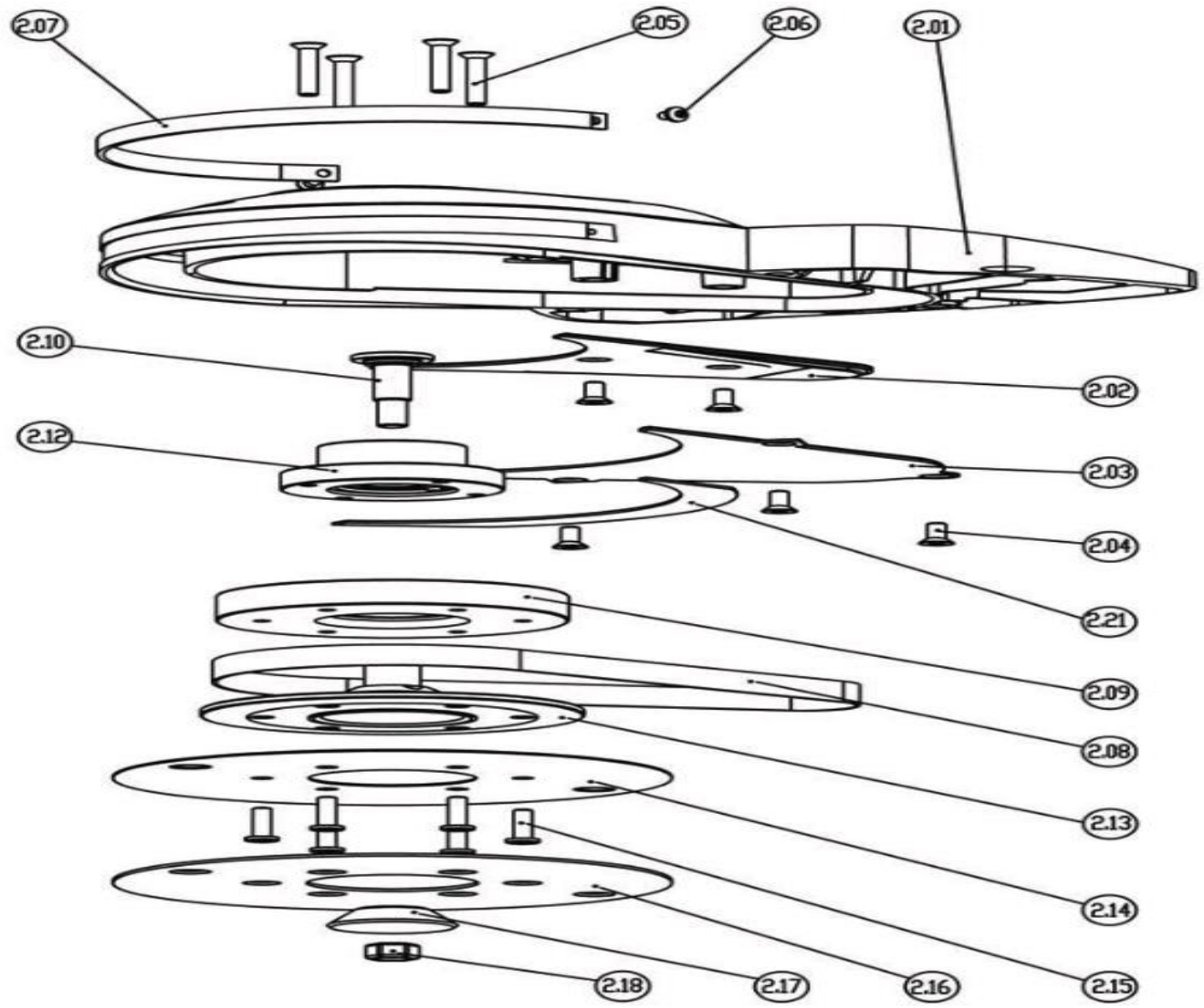
Bona Mini Edge AMO260001.0 Mini Edge sanding arm long
