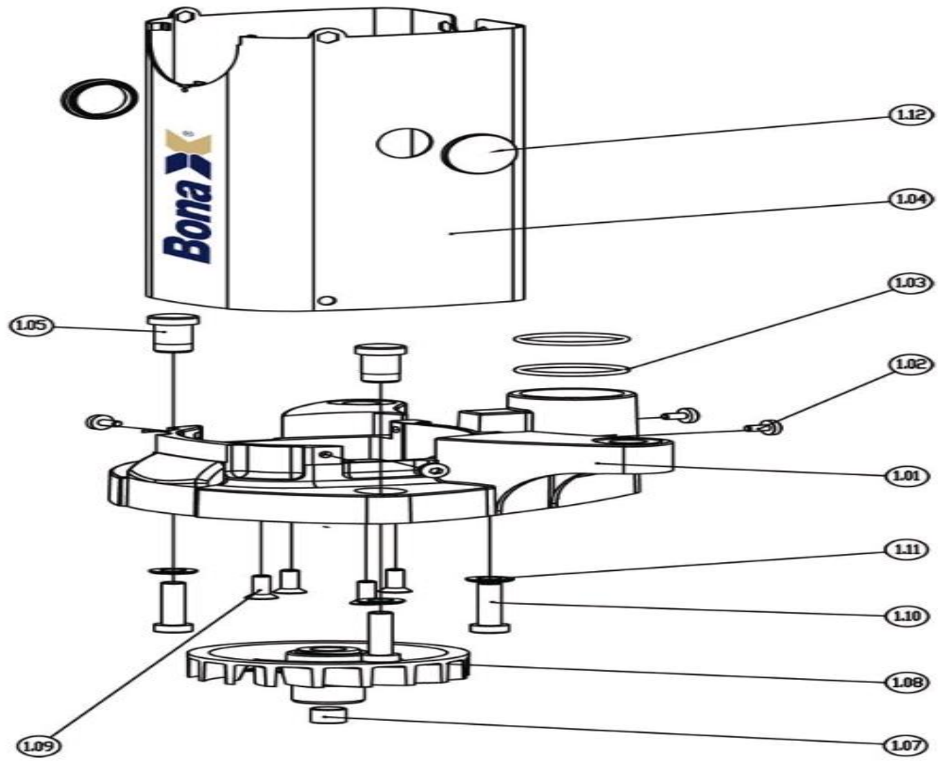
Bona Mini Edge AMO260001.0 Mini Edge Motor Bracket
