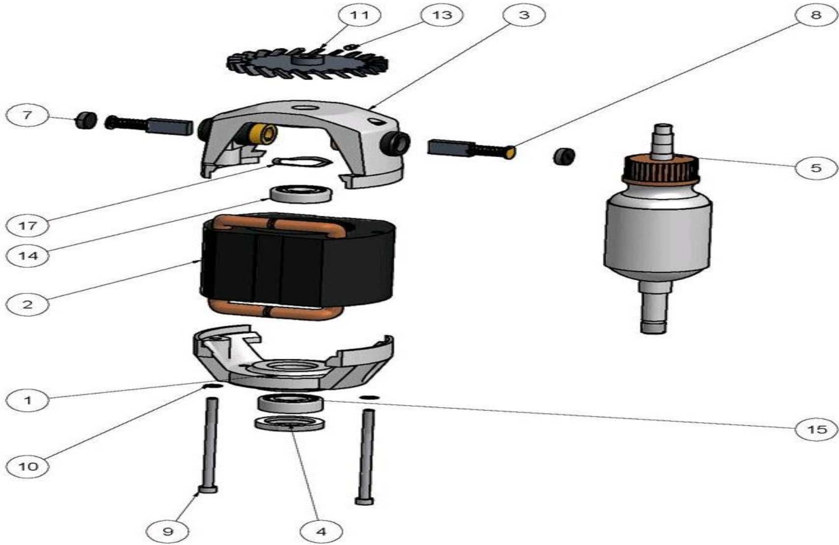
Bona Mini Edge AMO260000.3 Motor 1.3 kW 230V 50Hz ME
