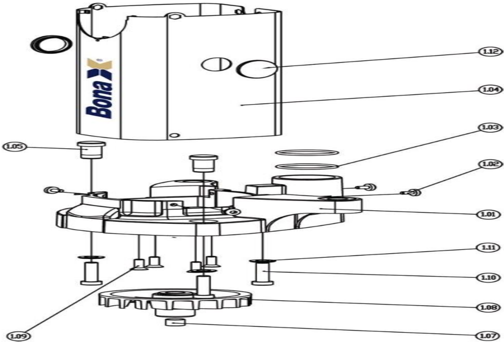
Bona Mini Edge AMO260000.3 Mini Edge Motor Bracket
