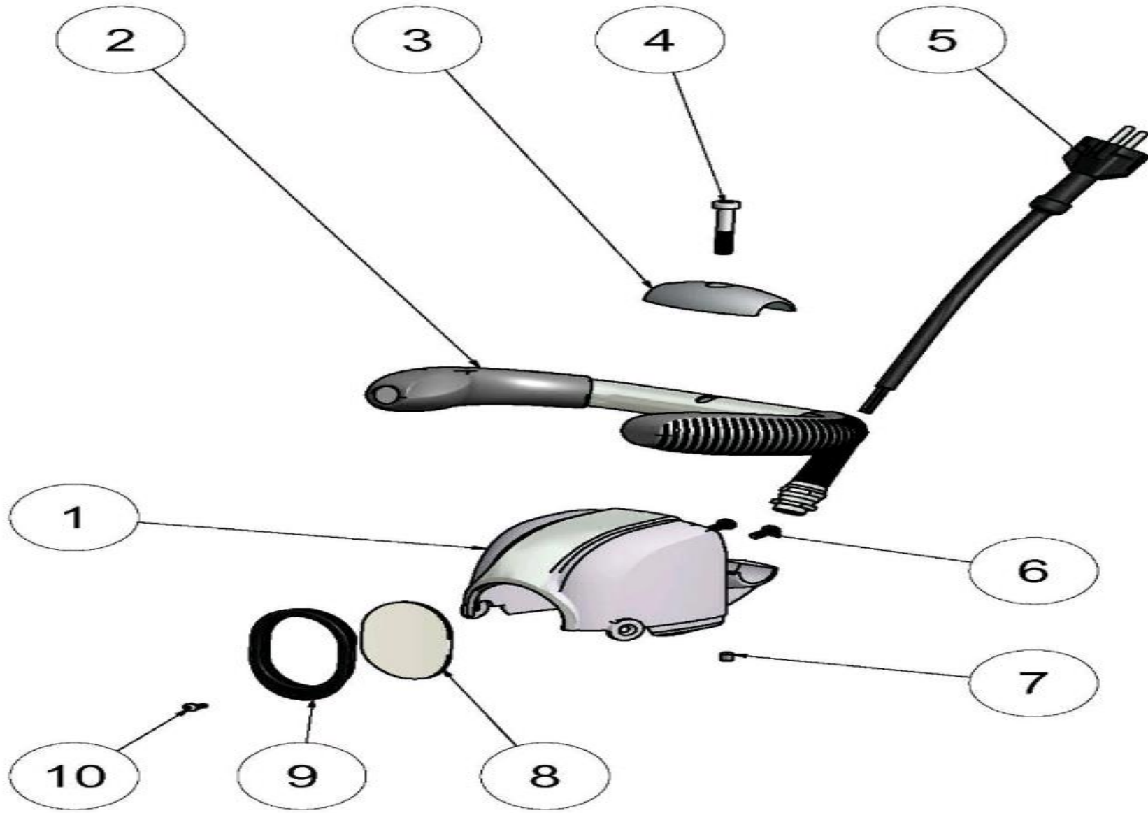
Bona Mini Edge AMO260000.3 Machine Cap 230V Basic
